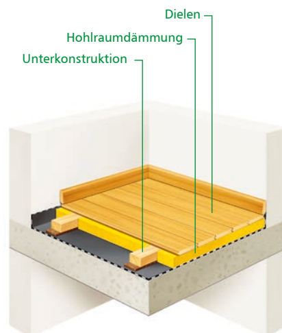
Dielenboden auf Stahlbetonplatte
